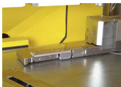
Längenmeßwagen Positioniergenauigkeit +/- 1 mm
